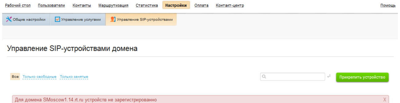
Рисунок 2 - Управление SIP-устройствами
