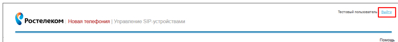
Рисунок 8 – Завершение работы
